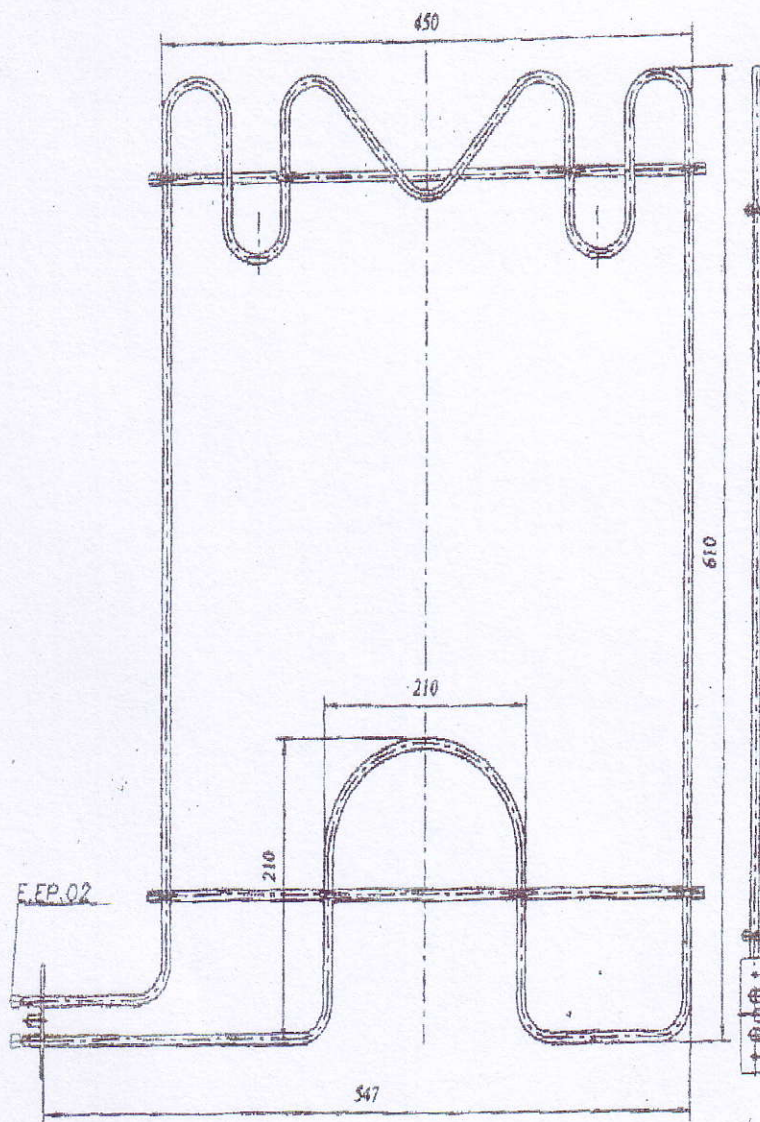
Слика 1 - Грејач печењаре „2500W“ - „IGO Ljubljana“
